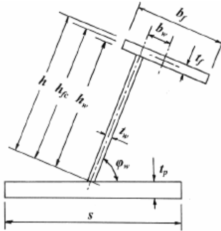
Fig. 4 Stiffener Geometry
